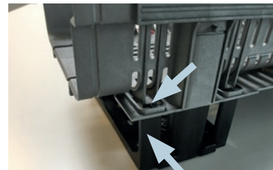
Die Verstelleinheit muss hier einrasten, ggf. seitlich ein wenig eindrücken.
