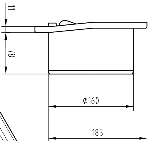
Stirnwand für Rinnenende mit Stützen DN/OD 160 Art.-Nr. 11094
