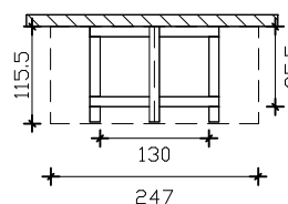
Grundrisse
