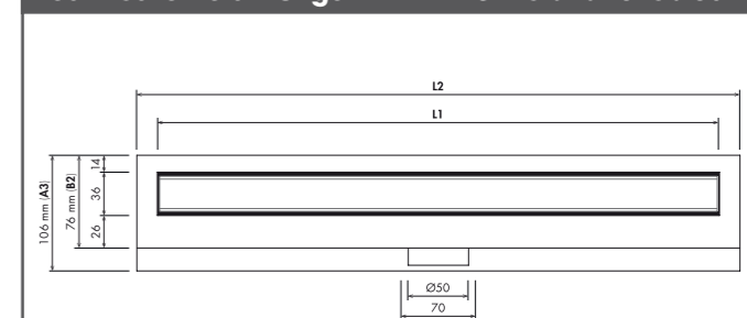
Draufsicht
