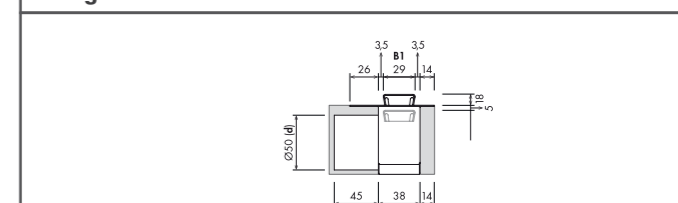
Seitenansicht
