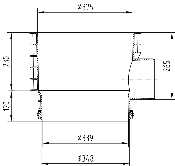
Schnitt A-A
