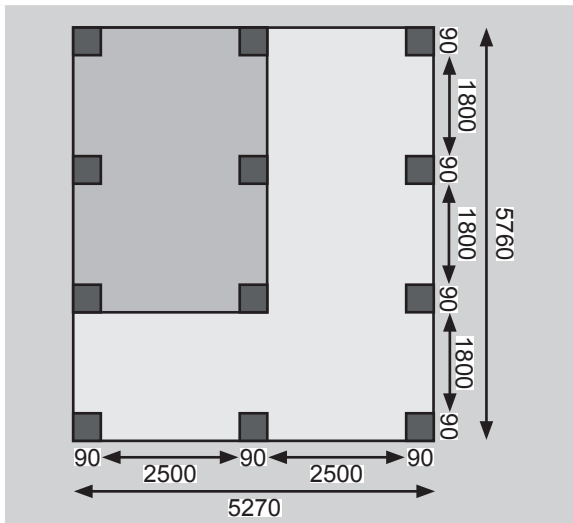
Carport + Abstellraum 2
