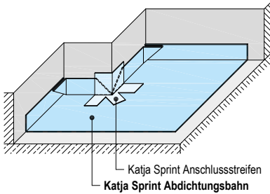
F457.de-P1 Vor- und rückspringende Ecken
