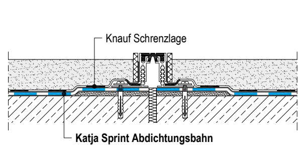
F457.de-V4 Estrich auf Trennschicht mit Schwerlastprofil
