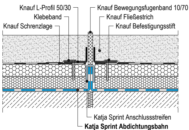
F457.de-V3 Estrich auf Dämmschicht
