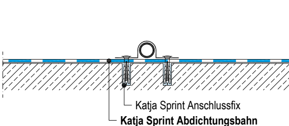
F457.de-V5 Rohrschelle auf Rohboden
