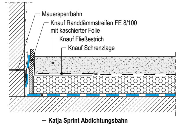
F457.de-V2 Mauersperrbahn auf der ersten Steinlage
