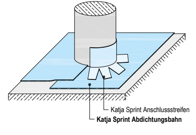
F457.de-P3 Runde Stützen
