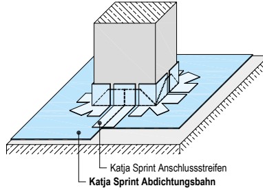
F457.de-P2 Rechteckige Stützen
