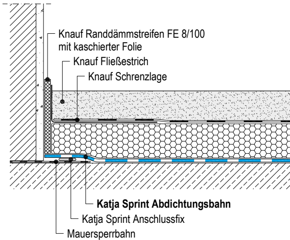
F457.de-V1 Mauersperrbahn auf der Bodenplatte
