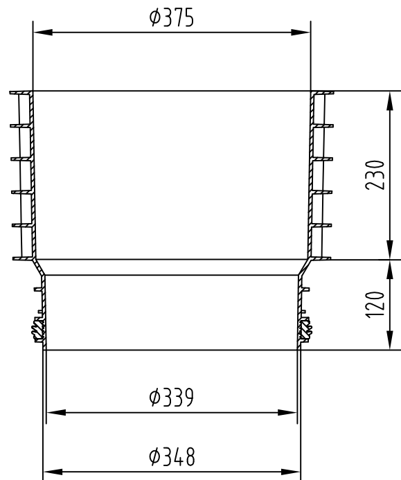
Schnitt A-A
