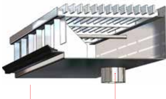
Anbindung und Entwässerung des Schwellsystems
