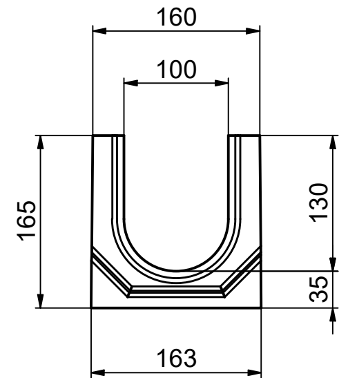
Ansicht Feder / view tongue / vue languette
