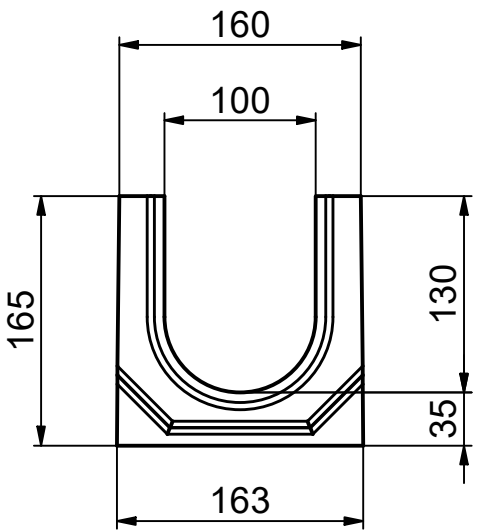
Ansicht Nut / view groove / vue rainure
