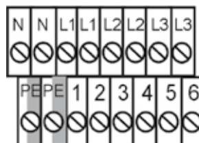
Anschluß Stromzuführung
