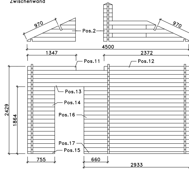
Zwischenwand
