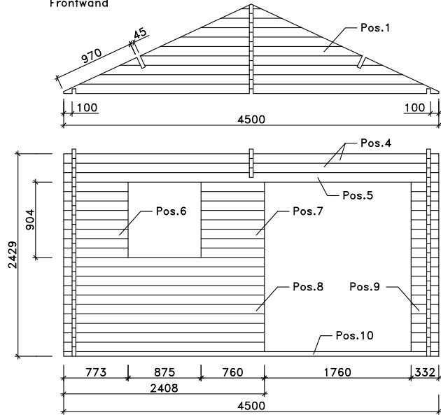
Frontwand
