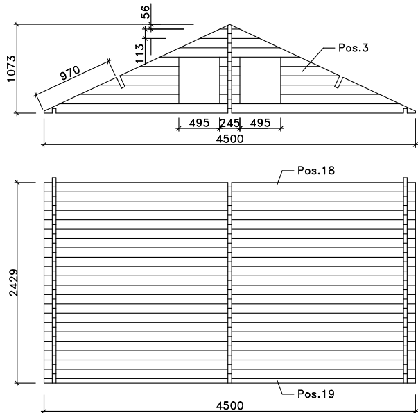
Rückwand
